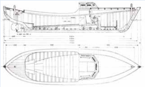
Tallinna-tüüpi mootorpaadi joonis.
